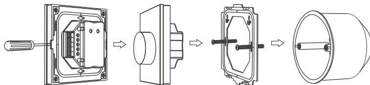
Рис. 4. Монтаж панели SMART
