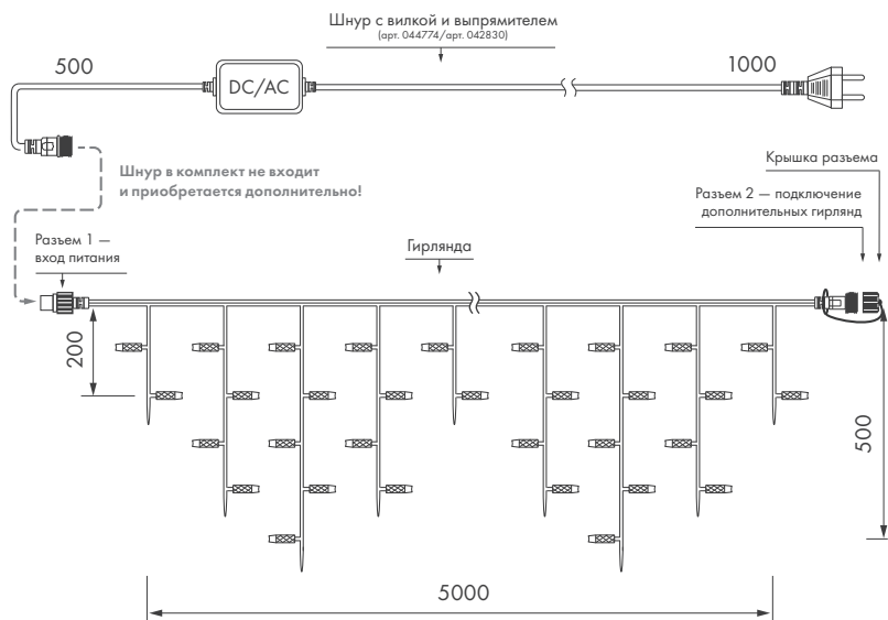
Рис. 1. Схема подключения гирлянды
