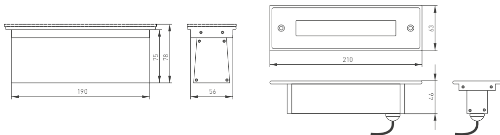
Рис. 1. Чертеж и габаритные размеры светильника
