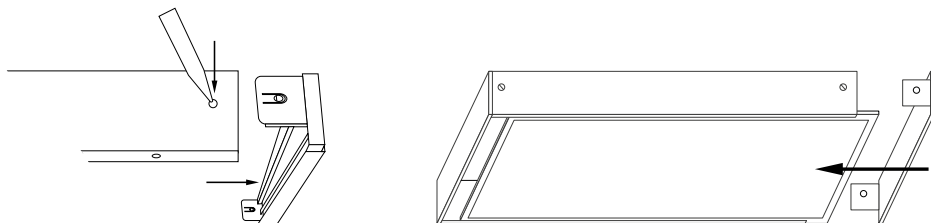
Рис. 3. Установка светильника
