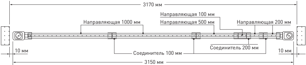
Рис. 3. Пример сборки направляющей длиной 3.15 м
