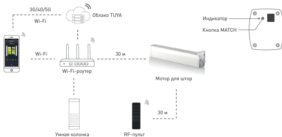
Рис. 6. Схема подключения электромотора с управлением TUYA
